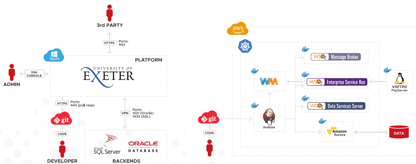
Esquema básico de la integración con WSO2
